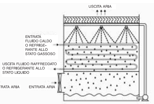
Figura 6 - Tiraggio forzato
